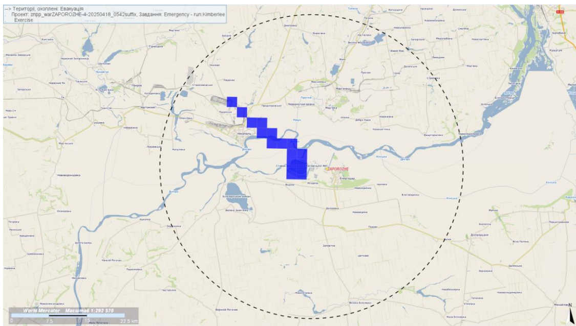
Рис.4. Результат моделювання просторового розподілу наслідків УРА на ЗАЕС (території, на яких рекомендована евакуація). Пунктиром позначено 30-ти кілометрову зону ЗАЕС. Розрахунок умовного викиду ЗАЕС з 09:00 (Київ) 18/04/2025
