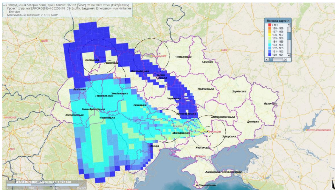
Рис.3. Результат моделювання просторового розподілу наслідків УРА на ЗАЕС (структура поля випадін довго існуючих радіоактивних елементів на прикладі Цезію-137). Щільність випадінь представлено у Бк/м². Розрахунок умовного викиду ЗАЕС з 09:00 (Київ) 18/04/2025
