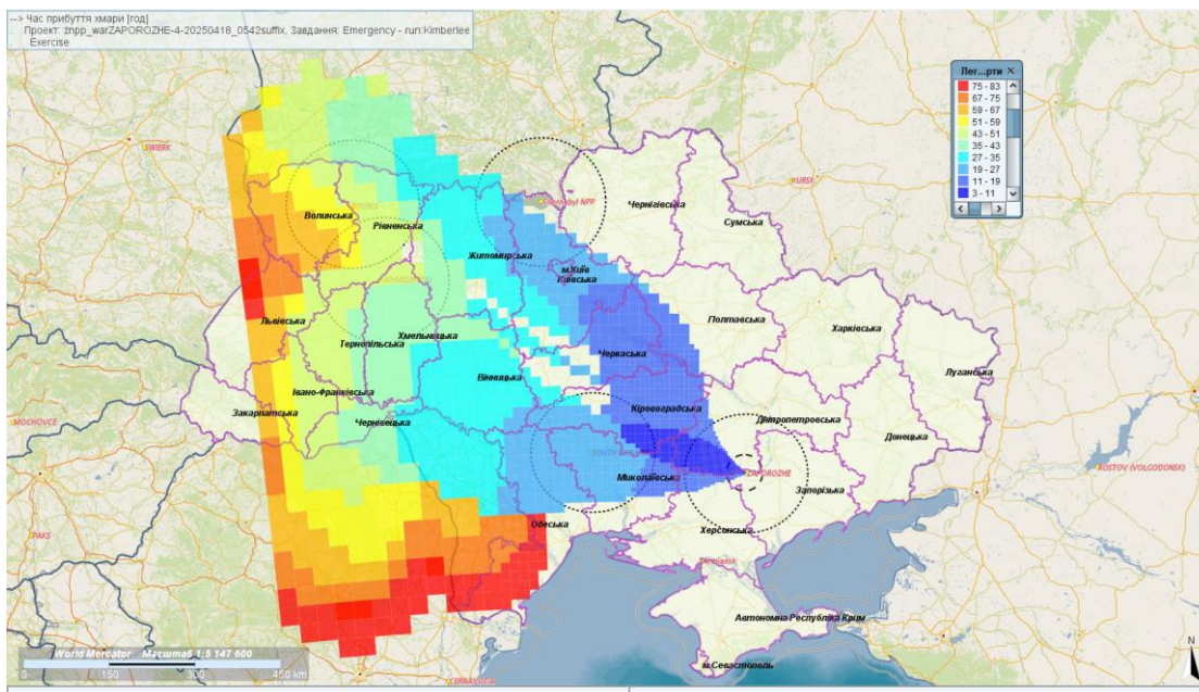
Рис.2. Прогноз поширення атмосферних мас з викидами ЗАЕС як наслідок УРА за 83 години. Час прибуття хмари. Швидкість поширення забруднення у годинах. Розрахунок умовного викиду з 09:00 (Київ) 18/04/2025. Тривалість умовного викиду 24 год.
