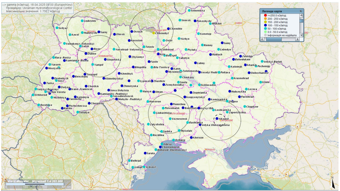
Рис.1. Радіаційний фон на території України за результатами спостережень мережі НГМС станом на 09:00 (Київ) 18/04/2025.
